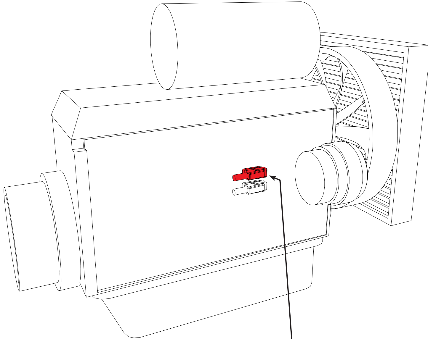
Original ECU Steckverbinder Original ECU connector
